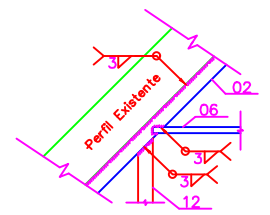
DETALHE 02 DETALHES DE SOLDA
