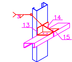
PERSPECTIVA LIGAÇÃO DAS TERÇAS
